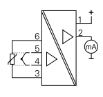
7501 HART Temperaturmessum- formen zur Feldmontage
