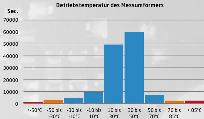
Beispiel für eine Erfassung interner Messumformertemperaturen
